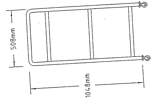
PANDANGAN SISI
