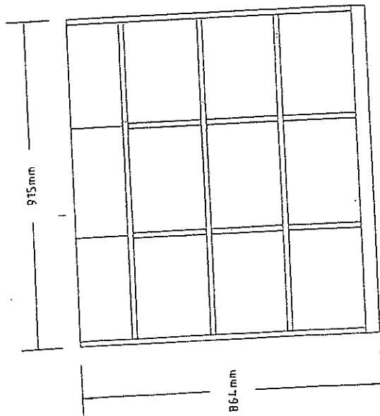
PANDANGAN DEPAN
