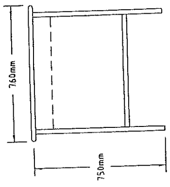
PANDANGAN SISI
