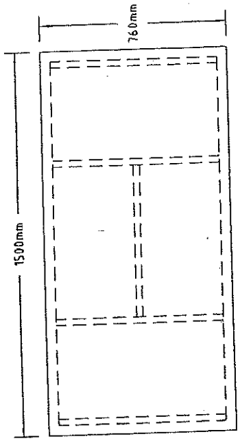
PANDANGAN ATAS
