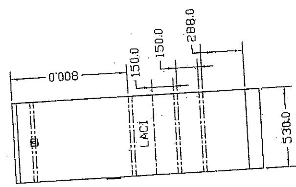
PANDANGAN SISI
