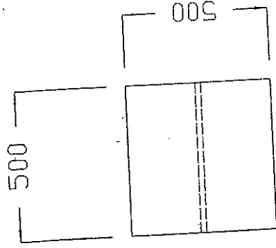
Pandangan Atas
