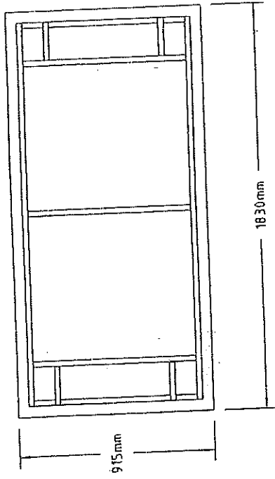
PANDANGAN ATAS
