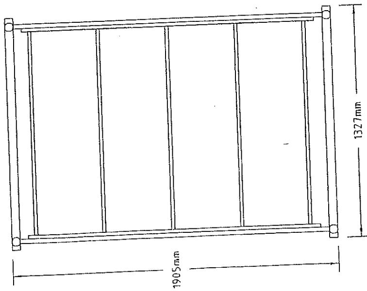
PANDANGAN ATAS
