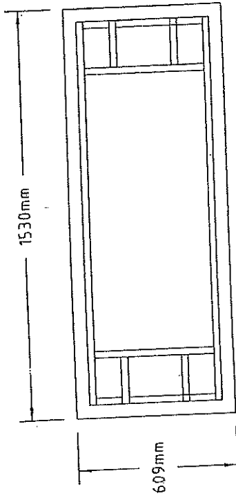
PANDANGAN ATAS
