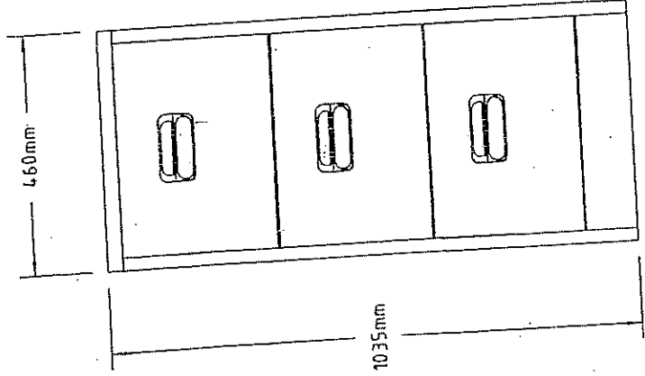
PANDANGAN DEPAN
