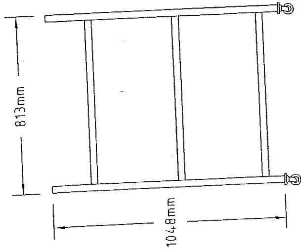
PANDANGAN DEPAN
